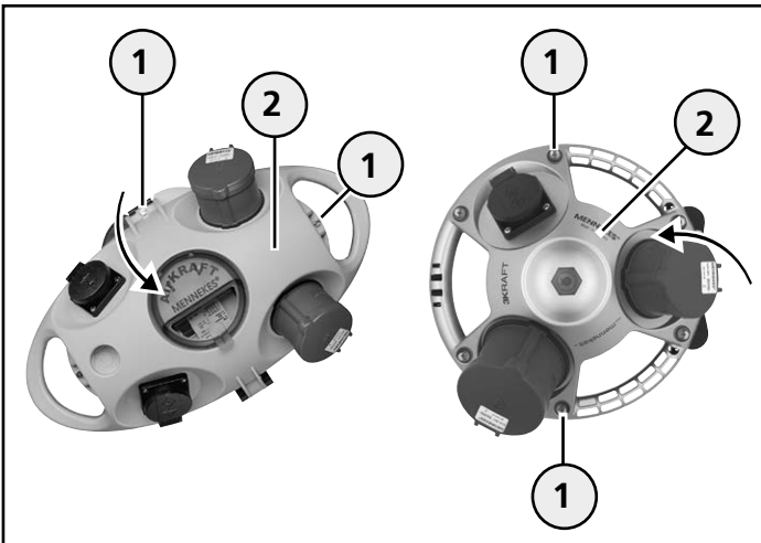
Ouverture de l'appareil
